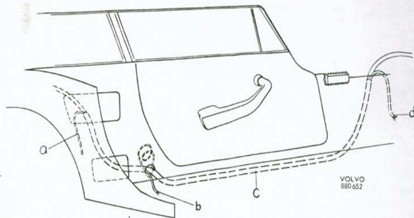
Fig. 4 Högtalarledningar
