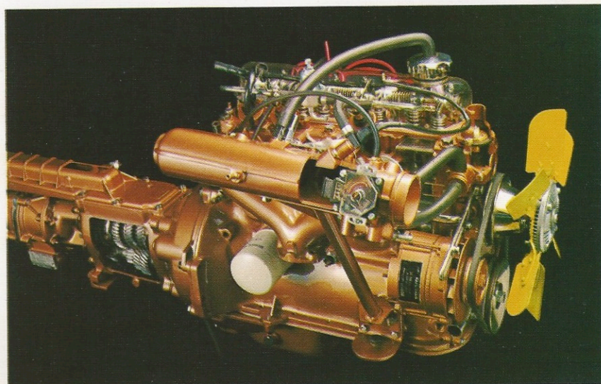
エンジンはB20E型の電子コントロール燃料噴射式、出力 135馬力(SAE)です。
