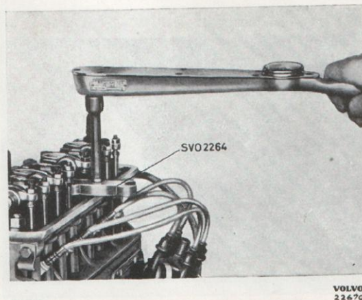
Bild 84. Efterdragning av cylinderlocksmuttrarna.
