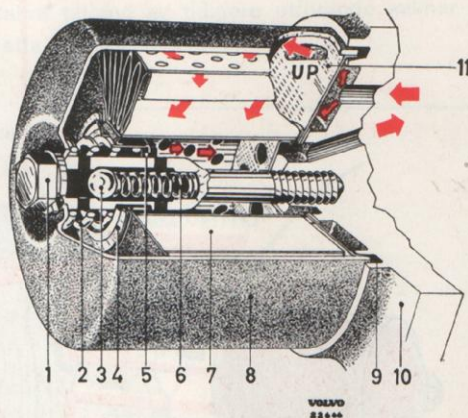
Bild 7. Oljerenare, Mann samt Fram.
