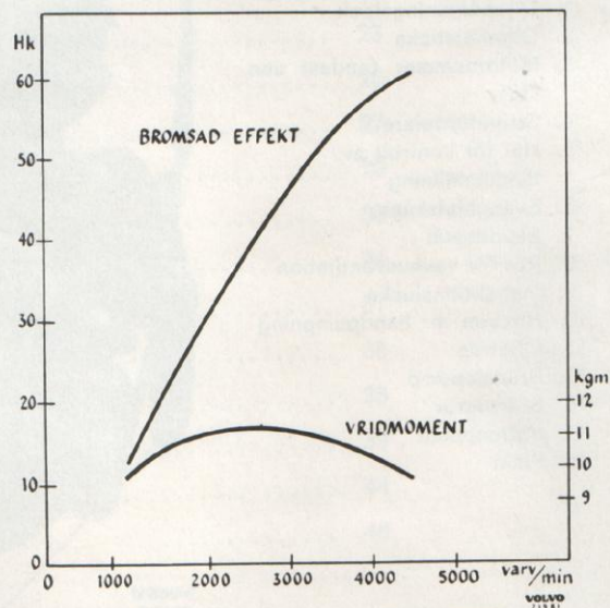
Bild 3. Effekt- och momentkurva (DIN).
