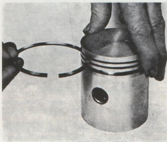
Bild 40. Kontroll av ringspel.
