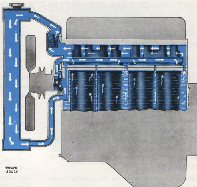
Bild 17. Kylsystem.
