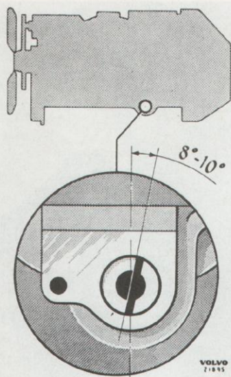
Bild 62. Pumpdrevets läge.
