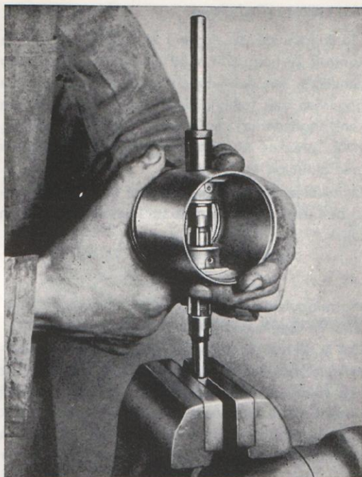
Bild 37. Brotschning av kolv.
