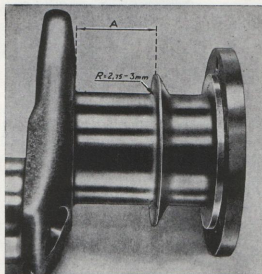
Bild 34. Styrlagertappens breddmått.
