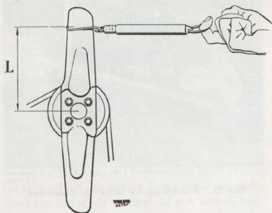
Bild 83. Remspänning.
