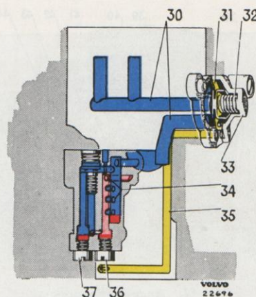
Bild 13. Munstycken och ekonomiventil.
