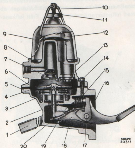
Bild 16. Bränslepump.
