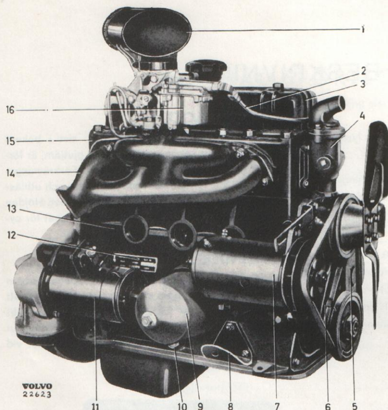
Bild 2. Motor från höger
