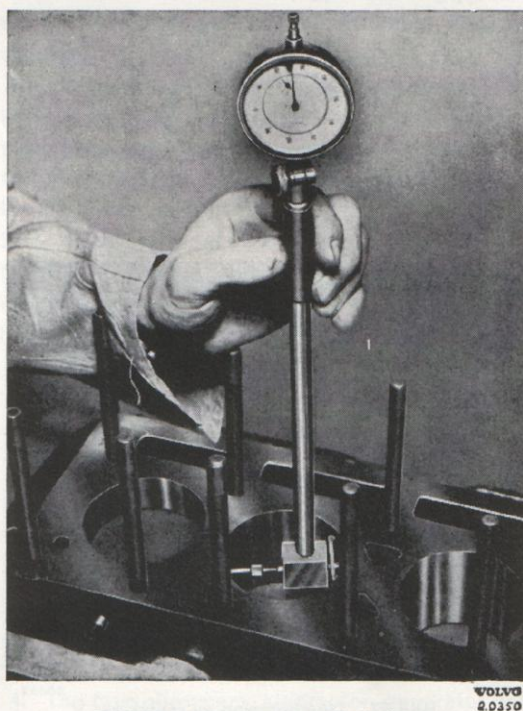
Bild 31. Mätning av cylinderlopp.
