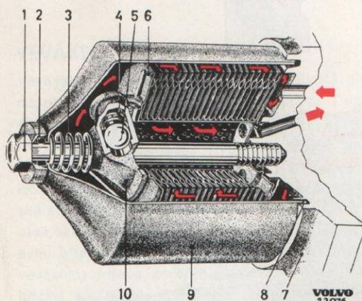
Bild 6. Oljerenare, AC.
