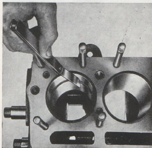
Bild 39. Kontroll av kolringens gap.
