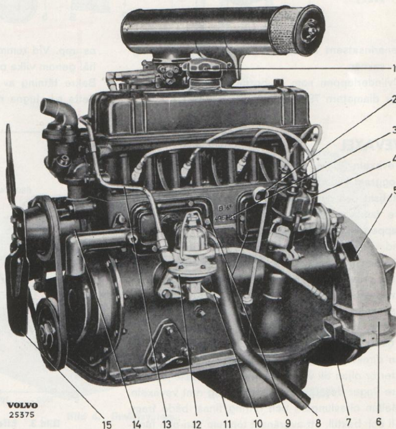
Bild 1. Motor från vänster.
