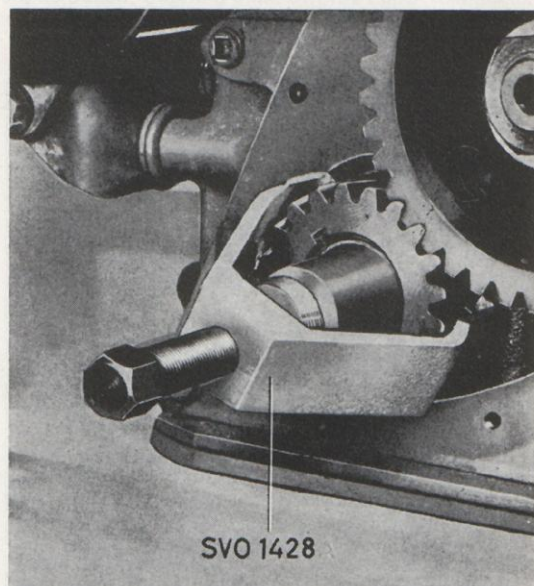
Bild 29. Demontering av vevaxeldrev.
