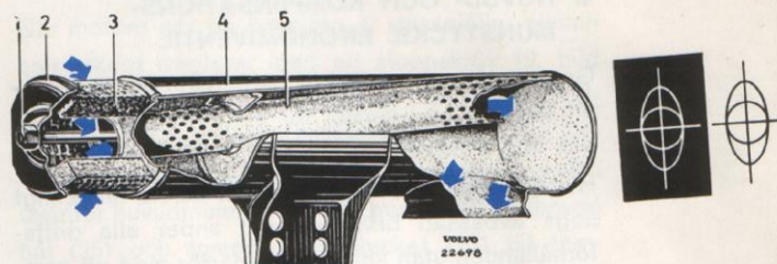
Bild 15. Luftrenare.
