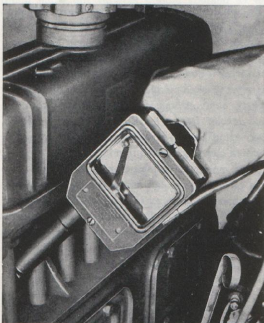
Bild 19. Kompressionsmätning.
