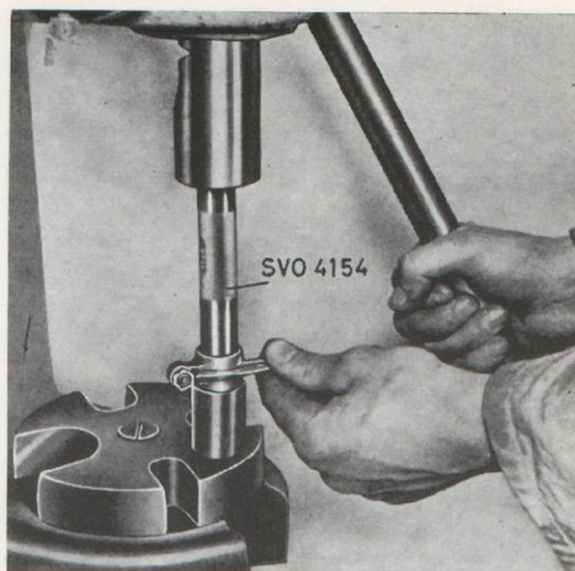
Bild 56. Byte av vipparbussning.
