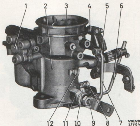
Bild 8. Förgasare från vänster
