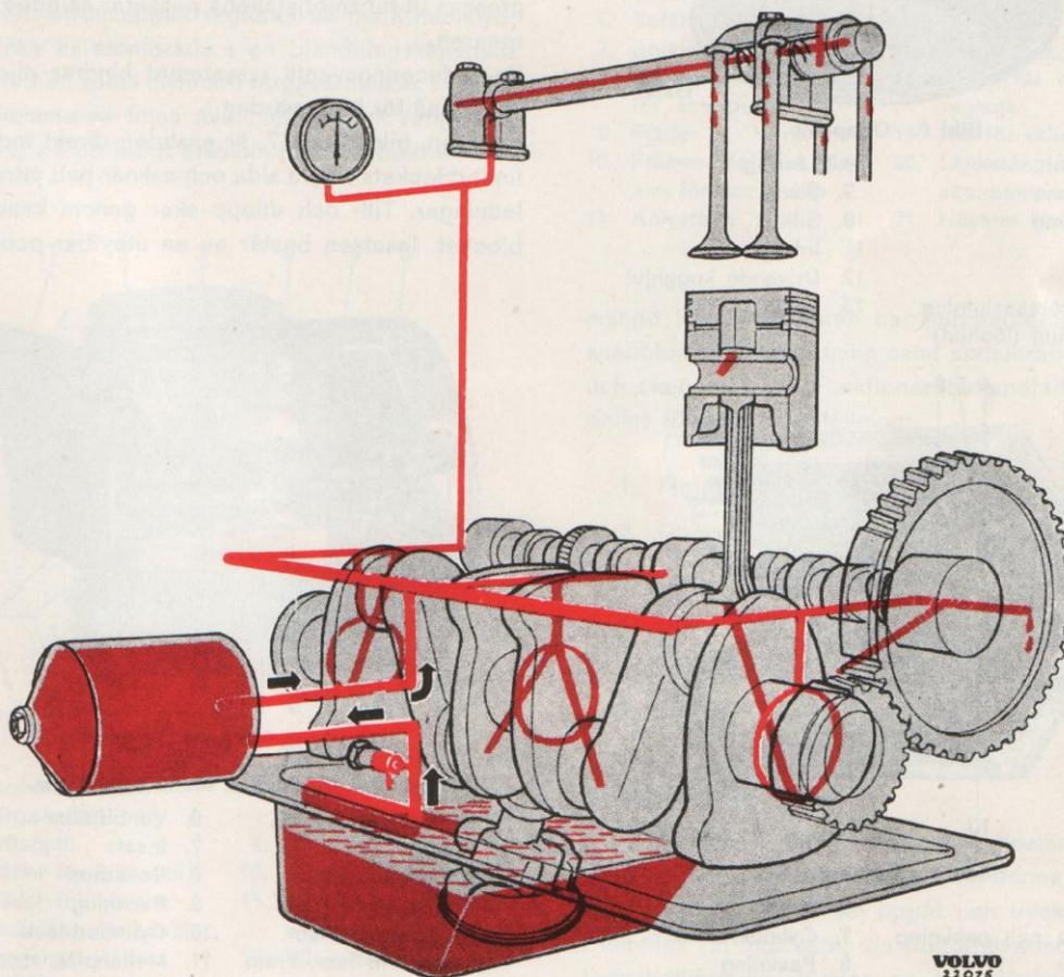
Bild 4. Smörjsystem.
