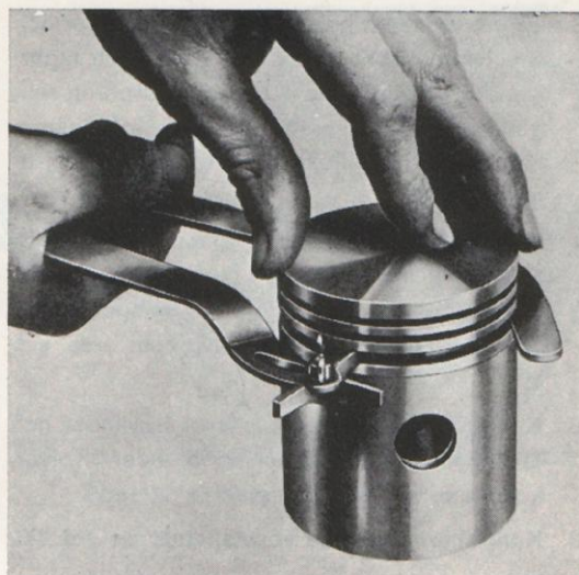
Bild 20. Rengöring av kolvringspår.
