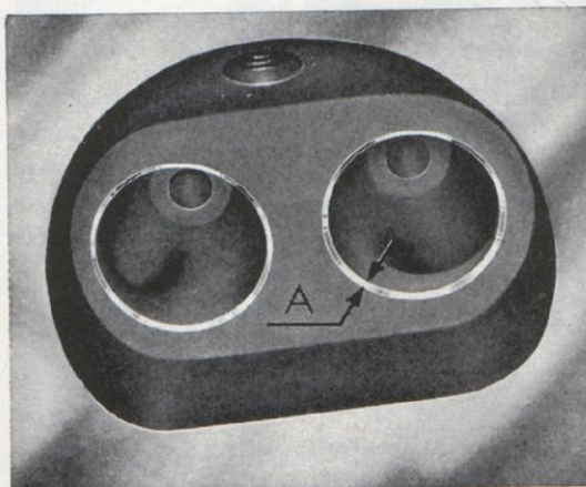
Bild 54. Ventil sätesbredd.
