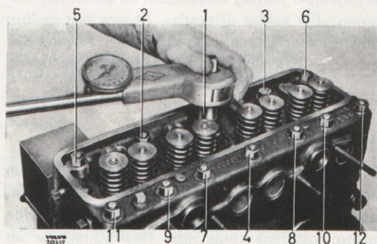
Bild 82. Åtdragningsföljd för cylinderlocksmuttrar.
