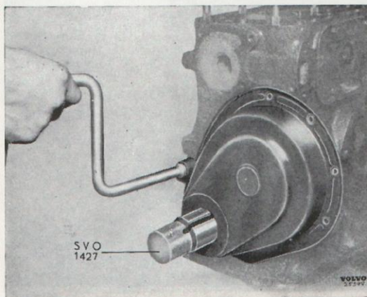
Bild 79. Montering av transmissionskäpa.
