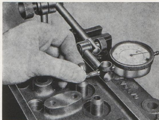
Bild 50. Mätning av spel.
