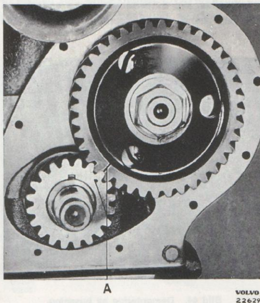
Bild 49. Inställning av transmissionshjulen.
