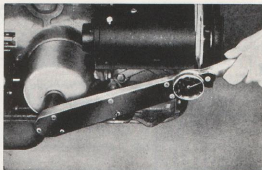
Bild 81. Åtdragning av skruv för oljerenerare.
