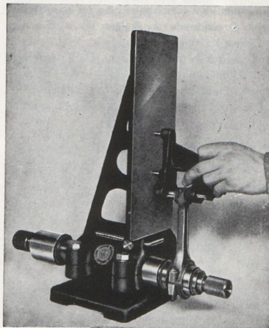
Bild 46. Indikering av vevstake.
