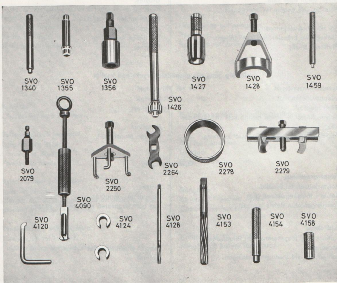
Bild 85. Verktug för motor.
