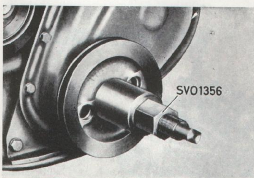
Bild 80. Montering av remskiva.
