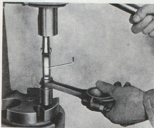
Bild 44. Demontering av bussning. 1. Dorn SVO 1355
