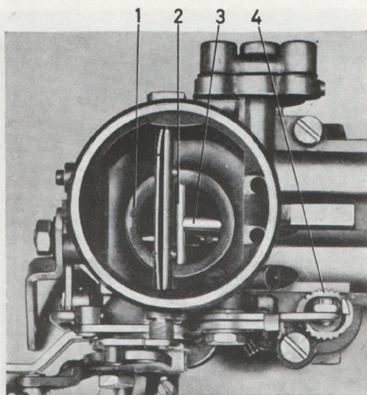
Bild 71. Luftkonans läge.
