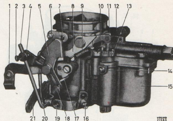
Bild 9. Förgasare från höger.
