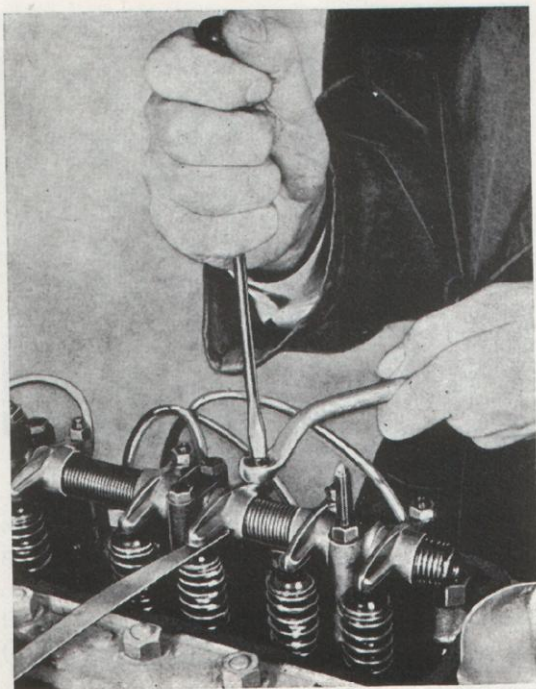
Bild 58. Justering av ventilspelet.
