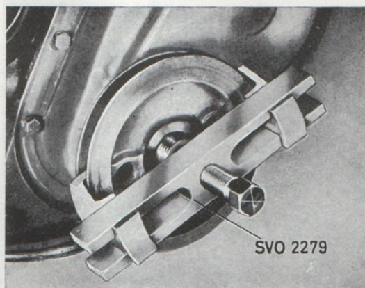
Bild 27. Demontering av remskiva.
