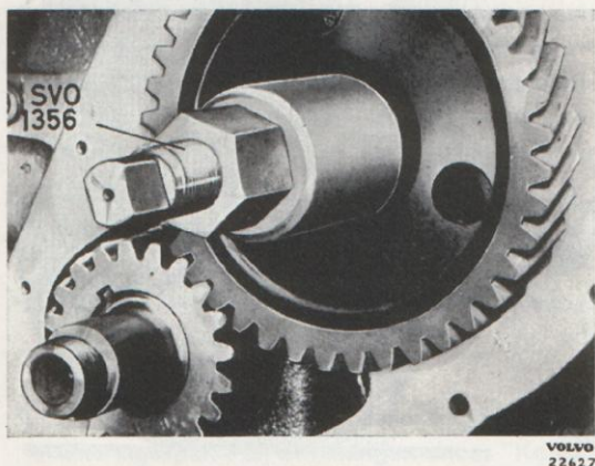
Bild 25. Montering av kamaxelhjul.
