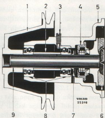
Bild 18. Vattenpump.
