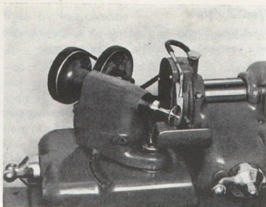
Bild 55. Ventilslipning.
