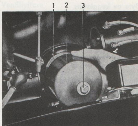
Bild 63. Byte av oljerenarens insats.
