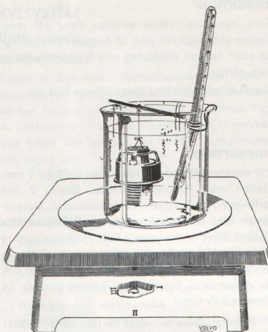
Bild 78. Provning av termostat.
