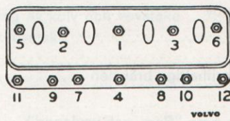
Bild 88. Åtdragningsföljd för cylinderlocksmuttrar.
