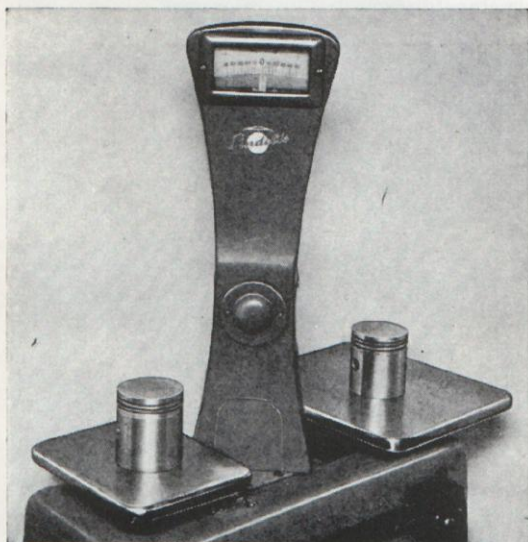
Bild 41. Vägning av kolvar.
