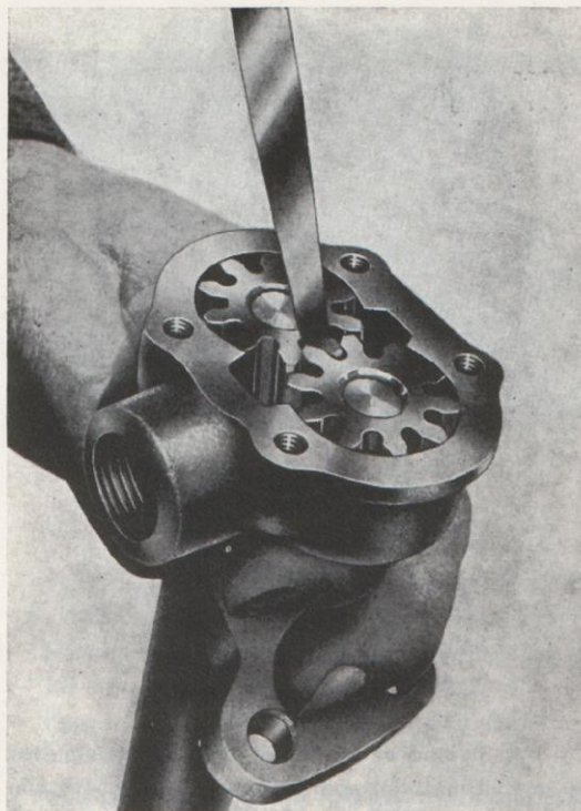
Bild 60. Mätning av kuggflankspel.
