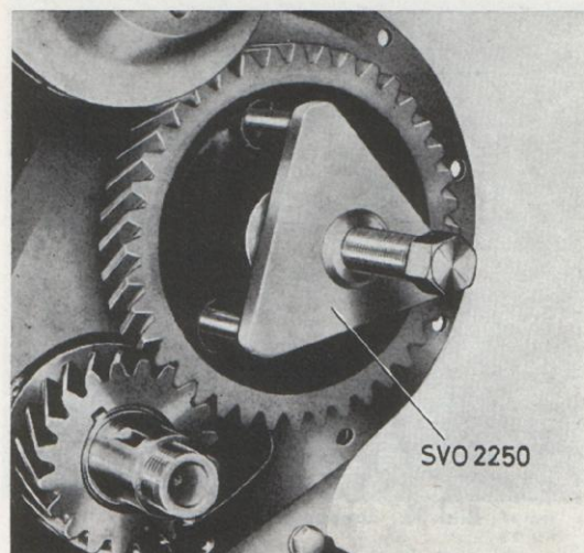
Bild 28. Demontering av kamaxelhjul.
