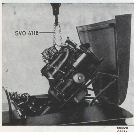
Bild 26. Demontering av motor.
