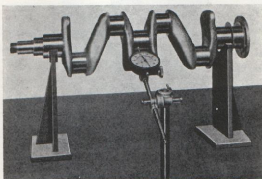
Bild 32. Indikering av vevaxel.
