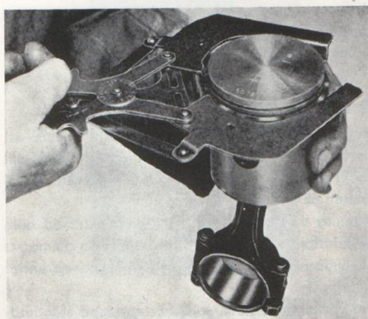
Bild 42. Montering av kolvringar.
