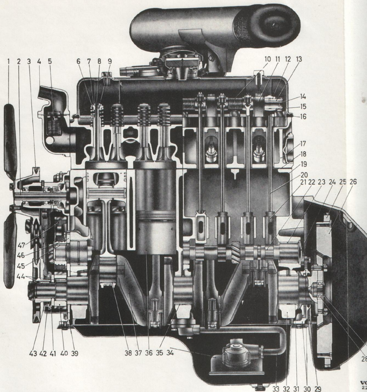
Plansch. Motor, B 16 A, längd- och tvärsnitt
