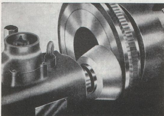
Bild 59. Planslipning av svänghjul.
