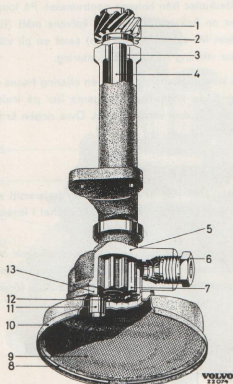
Bild 5. Oljepump.
