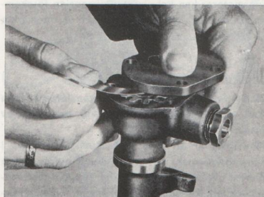
Bild 61. Mätning av axialspelet.
