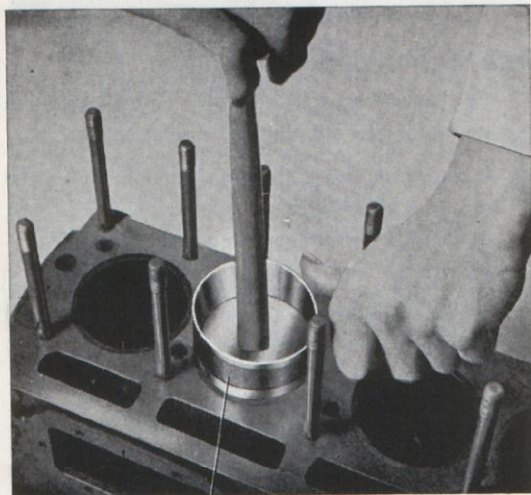
Bild 21. Montering av kolv. 1. SVO 2278
