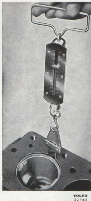
Bild 36. Mätning av kolvspel.
