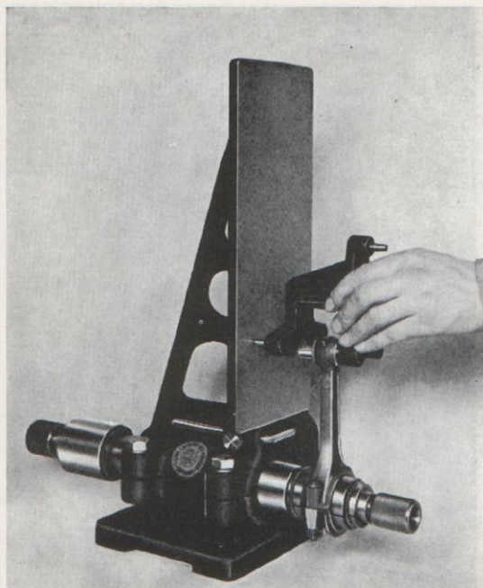
Bild 47. Indikering av vevstake.
