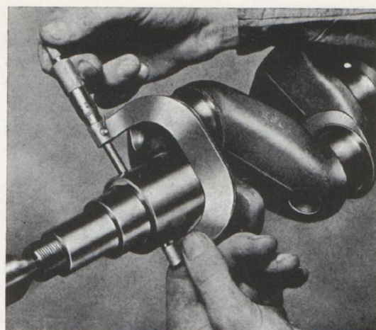
Bild 33. Mätning av lagertapp.
