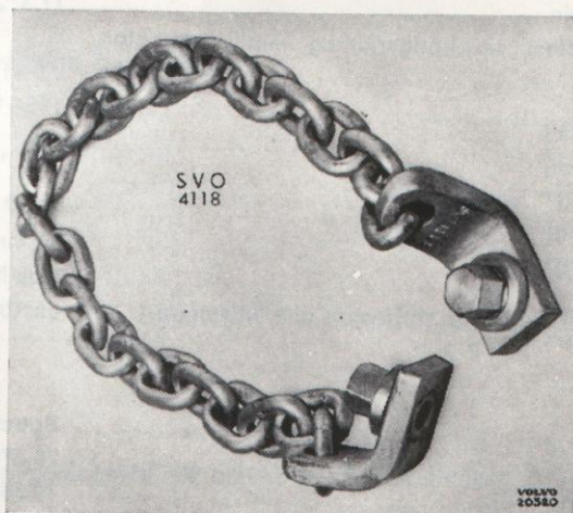
Bild 86. SVO 4118. Lyftkätting för motor.
